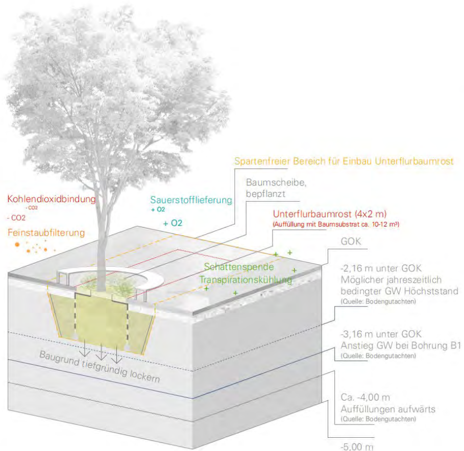
Unterflurbaumrost auf Betonfundament
